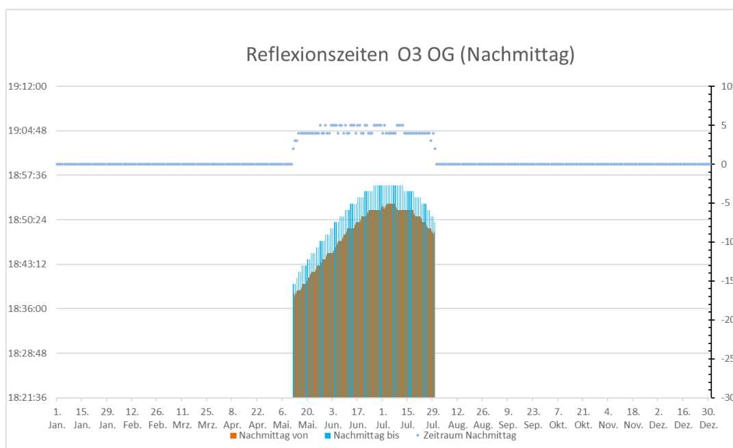
Abbildung 9: Reflexionszeiten und Dauer am Nachmittag zu Punkt O3 im OG
