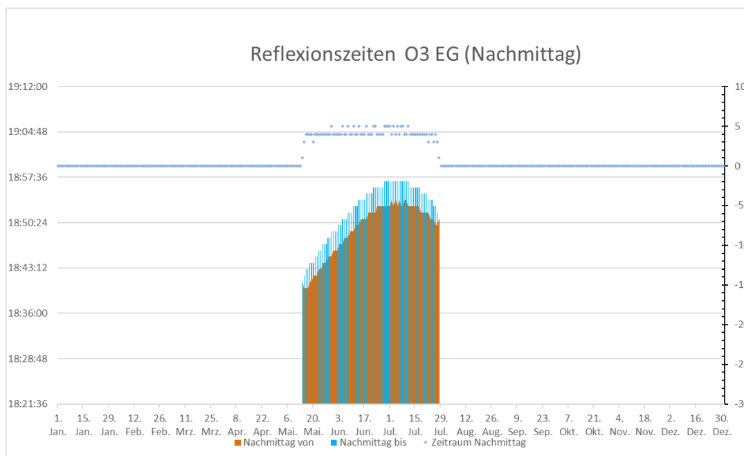
Abbildung 8: Reflexionszeiten und Dauer am Nachmittag zu Punkt O3 im EG
