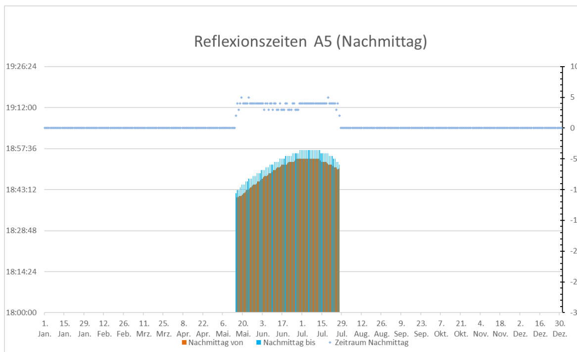
Abbildung 6: Reflexionszeiten und Dauer am Nachmittag zu Punkt A5
