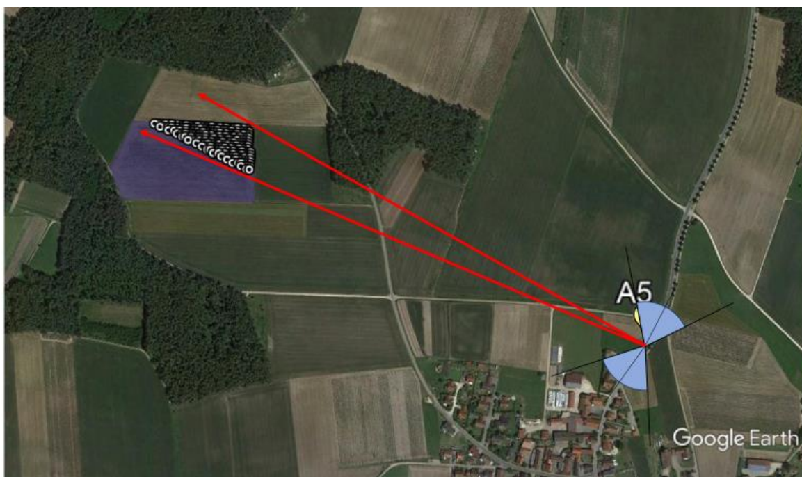
Abbildung 10: Vergleich Sichtfeld Fahrzeugführer für Punkt A5 mit Grenzvektoren in Richtung Module
